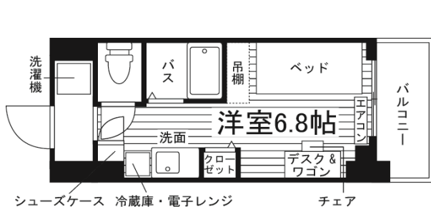
Aタイプ 1R (17.1㎡)
